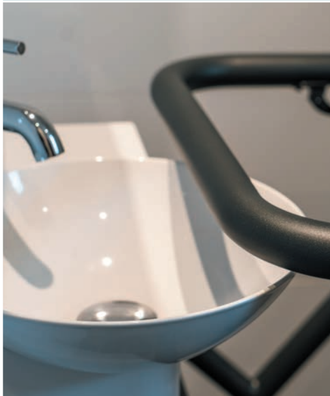
Null-Distanz-Funktion
